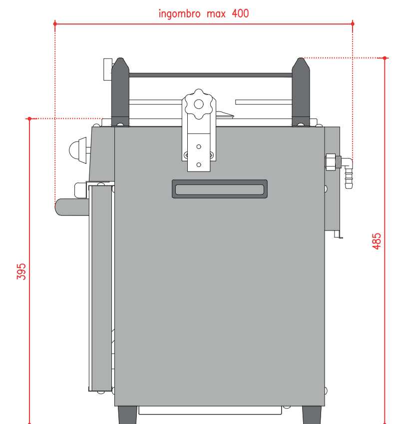
VISTA LATERALE SCALA 1:5
