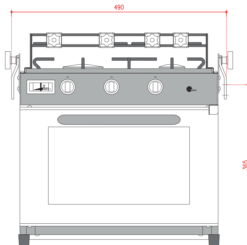
VISTA FRONTALE SCALA 1:5
