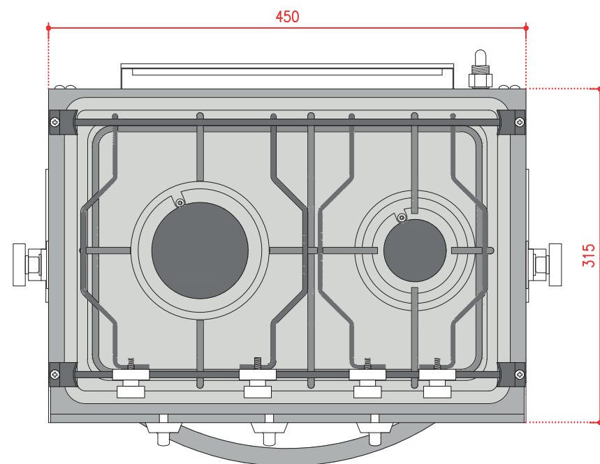
VISTA DALL'ALTO SCALA 1:5
